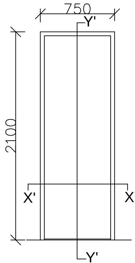
DOOR TYPE D3
